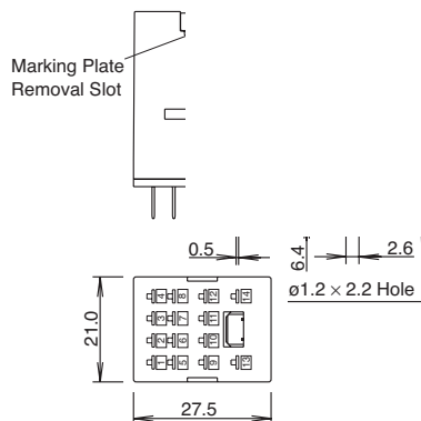
RU4S/RU42S
