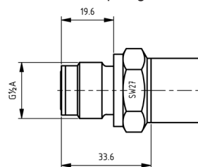
Fig. 4 - G 1/2 M, flush diaphragm
