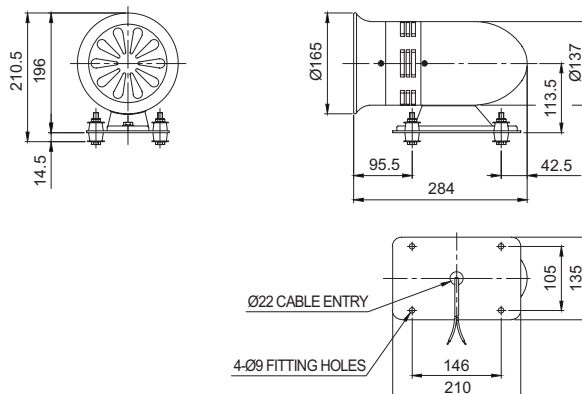
SM400
