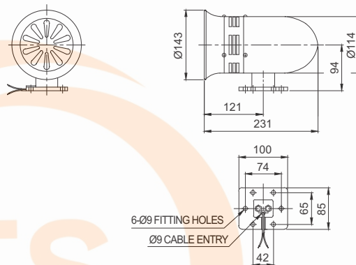
SM200
